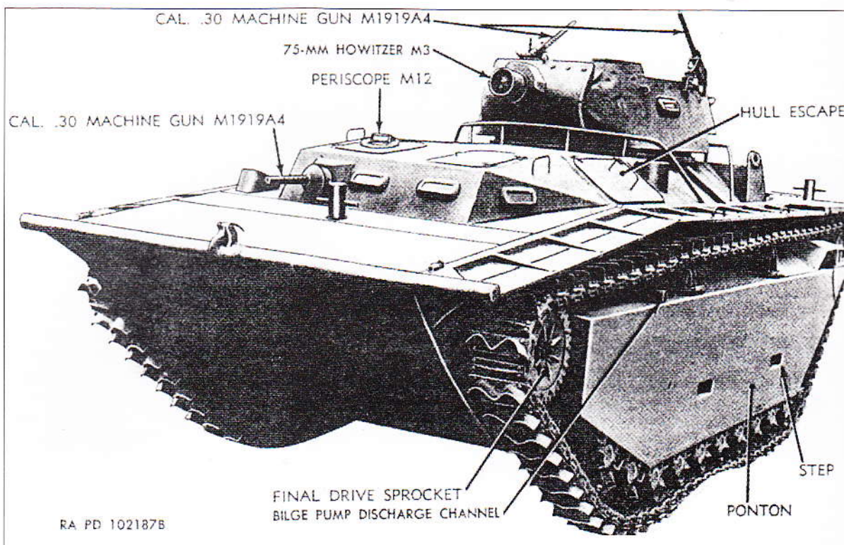
Плавающий танк LVT(A)-4 с двумя 7,62-мм пулеметами M1919A4 в кормовой части башни
