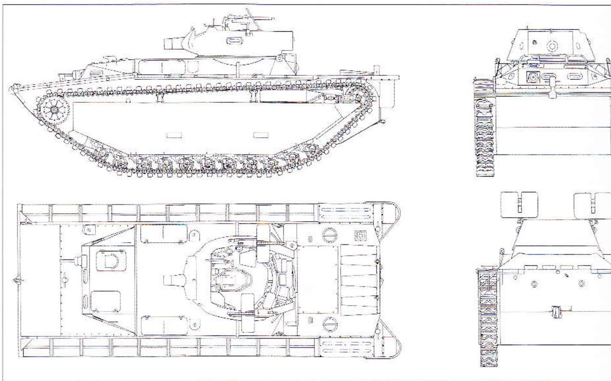
Проекция позднего варианта плавающего танка LVT(A)-4
